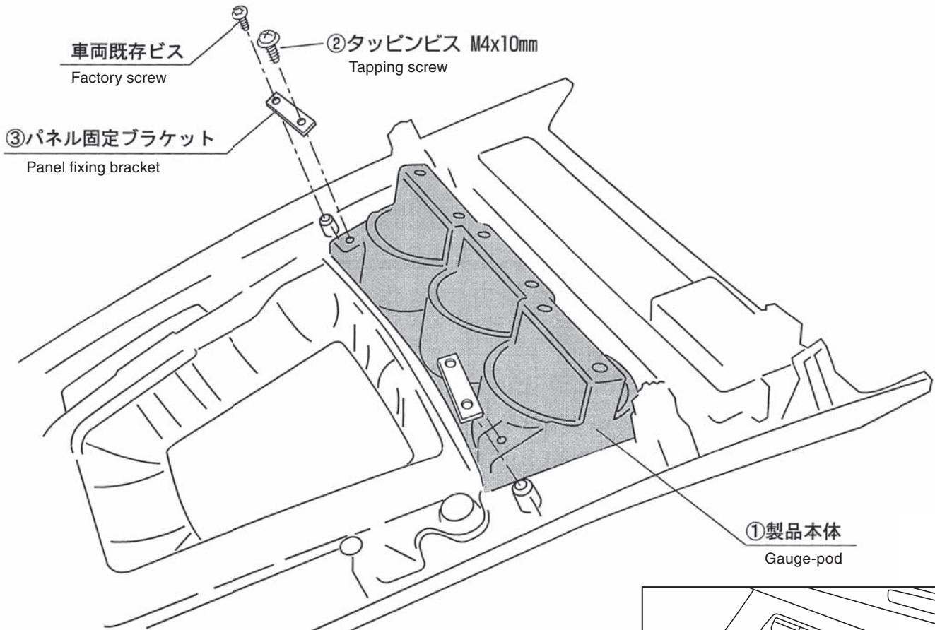
車両コンソールパネル（裏面） Car console panel (back side)
